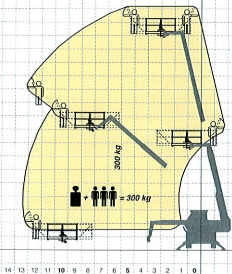
ROTO 38.16 / ROTO 38.16 S PLATEFORME PORTE-PERSONNES SUR 360°
