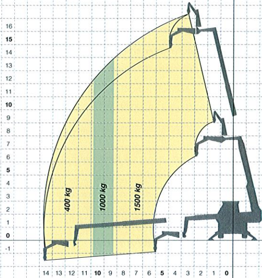
ROTO 38.16 / ROTO 38.16 S FLECHETTE AVEC TREUIL SUR 360°
