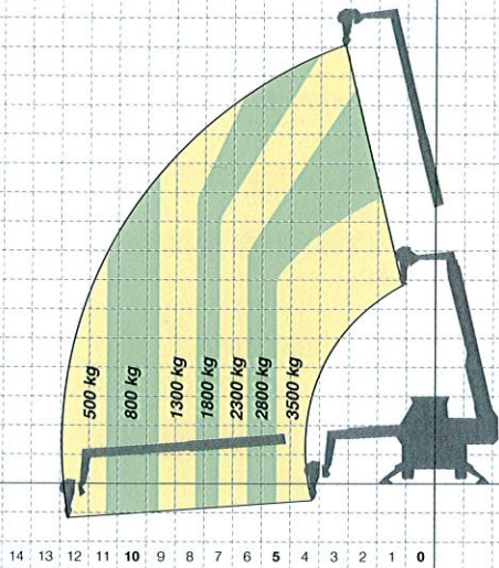
ROTO 38.16 / ROTO 38.16 S TREUIL SUR 360°
