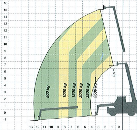
ROTO 38.16 S FOURCHES SUR PNEUS - FRONTAL
