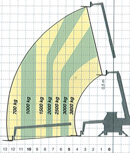
ROTO 38.16 / ROTO 38.16 S FOURCHES SUR STABILISATEURS SUR 360°
