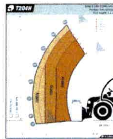
Tablier Universal
